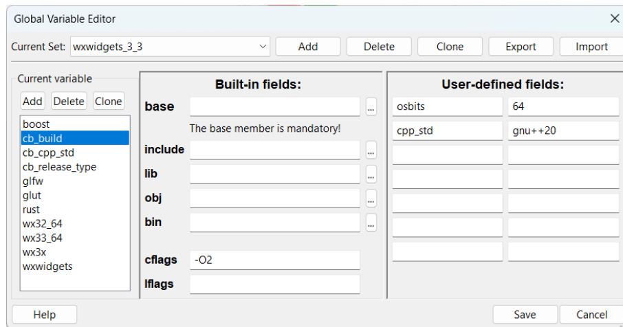
Figure 6.2: Configuration pour générer CB
