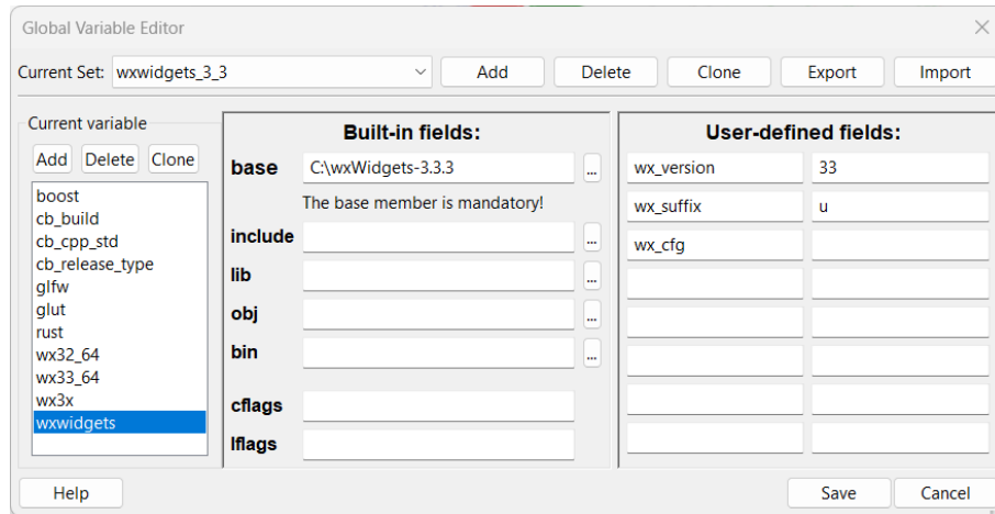
Figure 6.4: Configuration de la variable wxwidgets avec un champ vide
