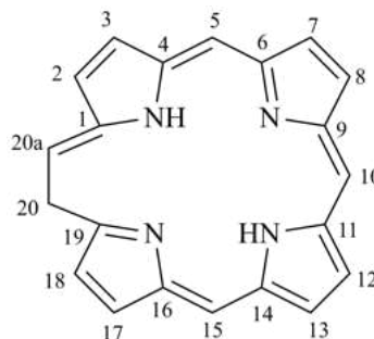
(B) 20H-20a-homoporphyrin
