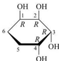
(1 R ,2 R ,3 R ,4 R )-cyclohexane-1,2,3,4-tetrol
