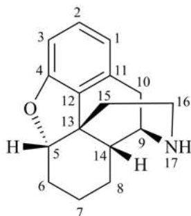
4,5 \alpha -epoxymorphinan
