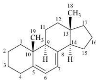
androsta-5,7-diene
