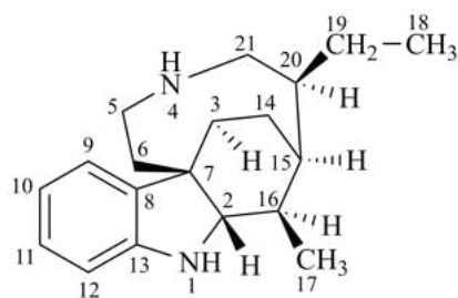
3,4-secocuran
