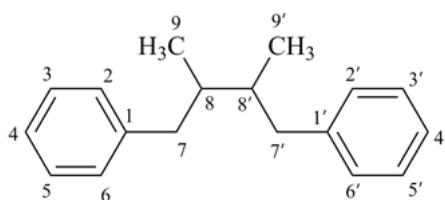
lignane
