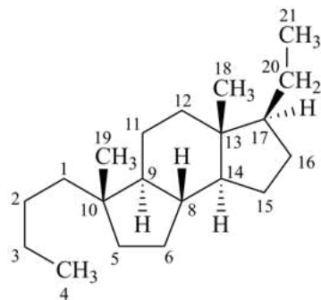
4,5-seco-7-norpregnane
