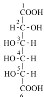
L-altritic acid (not L-talaric acid)
