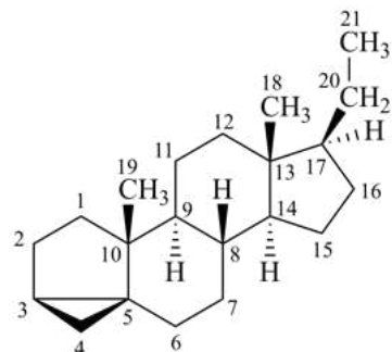
3 \alpha ,5-cyclo-5 \alpha -pregnane
