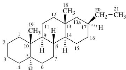
13(17)a-homo-5 \alpha -pregnane
